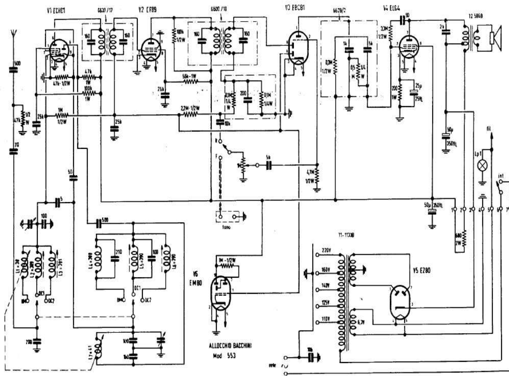
Schema elettrico del radioricevitore Allochio Bacchini, mod. 553
